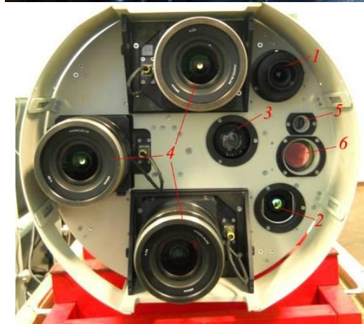
Общий вид
